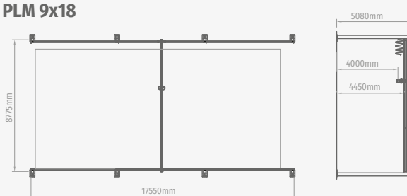
PLM 9x18
